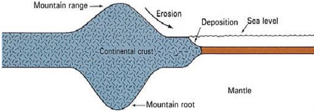
চিত্র-৩: মাটির ভিতর গভীর শিকড় থাকার কারণে পাহাড় কিভাবে পেরেকের মত রূপ নিয়েছে চিত্রটি তা ব্যাখ্যা করছে। (Earth Science, Tarbuck and Lutgens)
