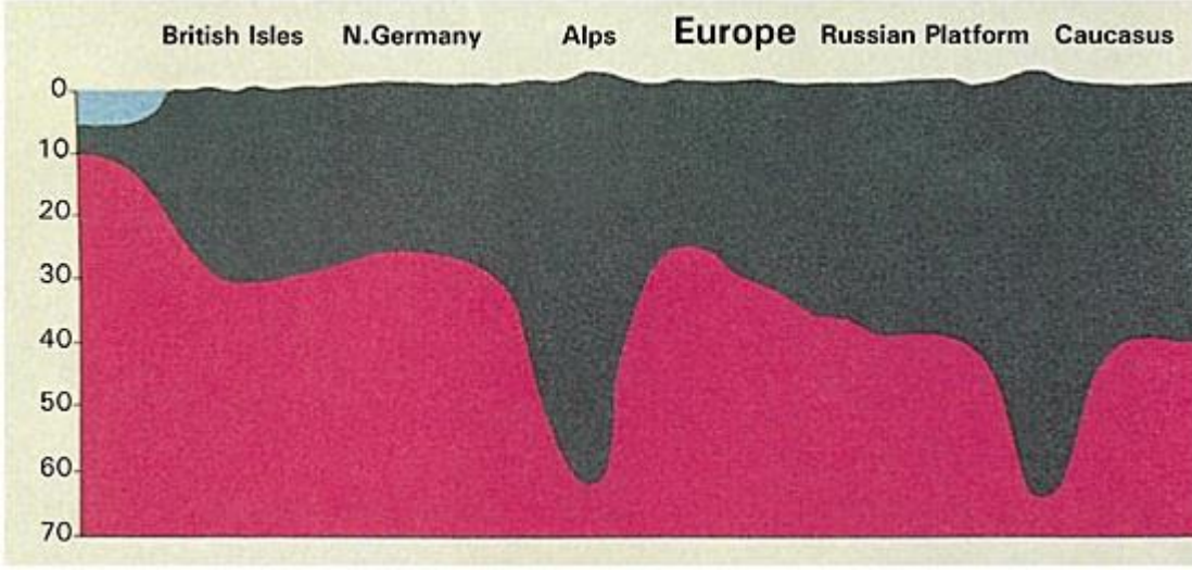
চিত্র-২: চিত্রে পাহাড়কে পেরেকের মত দেখা যাচ্ছে মাটির গভীরে যার রয়েছে প্রোথিত শিকড়। (Anatomy of the Earth, ২২০ পৃষ্ঠা)
